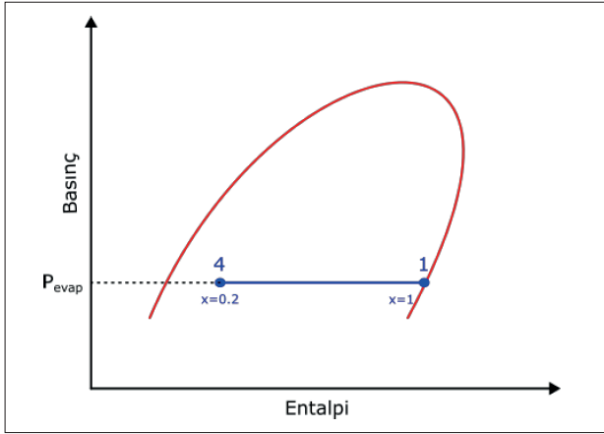
Şekil 1. P-h diyagramı
