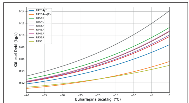
Şekil 2. Soğutucu akışkanların kütleli debi-buharlaşma sıcaklığı grafiği.
