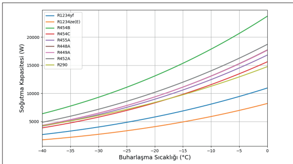
Şekil 3. Soğutma kapasitesi-buharlaşma sıcaklığı grafiği
