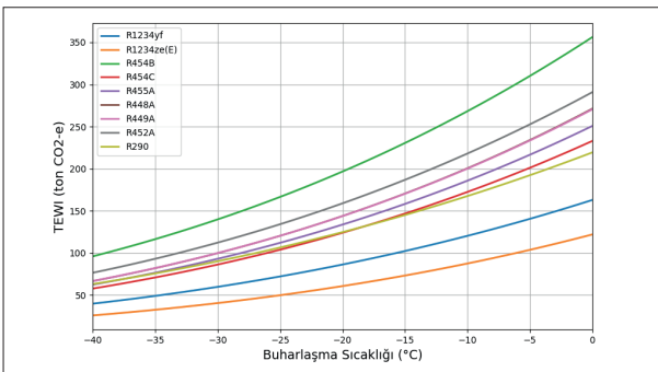
Şekil 4. TEWI değerleri
